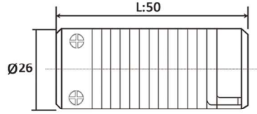
MEKANİK ÖLÇÜLER
